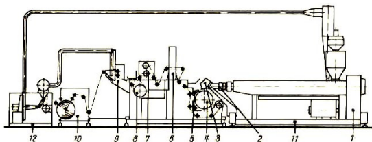
Bild 1. Schematische Darstellung einer Breitschitz-Flachfolienanlage
